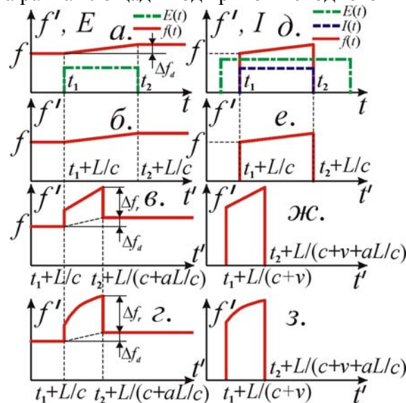
Рис. 6. Преобразование частоты излучения в трансформаторе Ритца. Слева – для непрерывного излучения + импульсы напряжения E(t) . а) начальный сигнал сразу после переизлучения, б) на расстоянии r по СТО, в) на расстоянии r по БТР, г) то же при v \sim c и f\Delta t \sim c . Справа – то же, но для импульсного излучения. д) Начальный сигнал, е) на расстоянии r по СТО, ж) на расстоянии r по БТР, з) то же в релятивистском случае, при v \sim c и f\Delta t \sim c .
