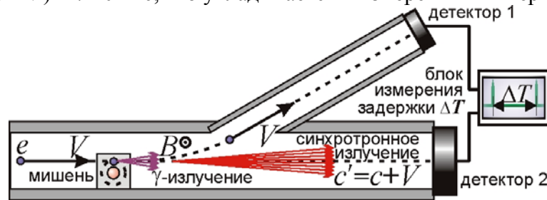
Рис. 9. Схема опыта Брауна.
