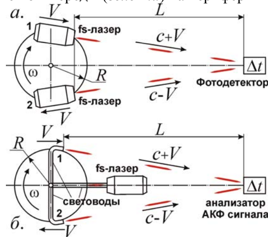
Рис. 1. Схемы установок по сравнению скоростей света от движущихся источников.
